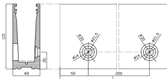
Perfil U 54300-MF03
