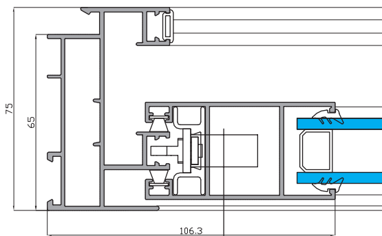
Sección Horizontal
