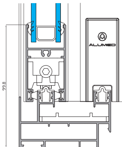
Sección Vertical
