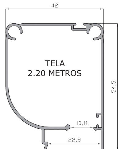
Cajón Mosquitera terminal tela 2.20 metros 31005
