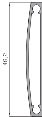
Travesaño mosquitera Curvo 99011
