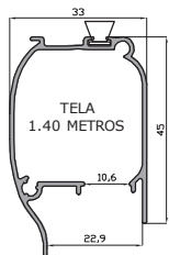
Cajón Mosquitera terminal tela 1.40 metros 31006
