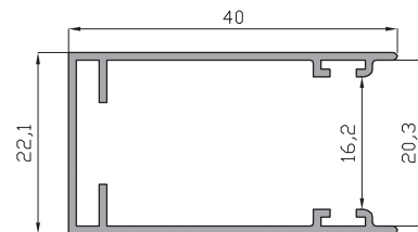
Guia lateral doble felpa 31002
