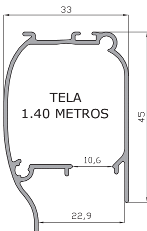
Cajón Mosquitera terminal tela 1.40 metros 31006
