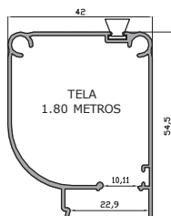
Cajón Mosquitera terminal tela 1.80 metros 31001
