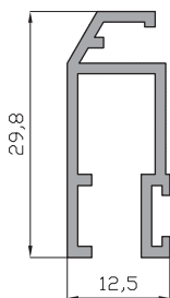
Hoja perfil mosquitera 54572
