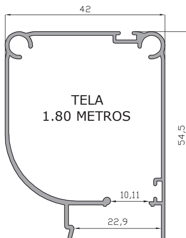
Cajón Mosquitera terminal tela 1.80 metros 31001
