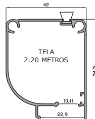
Cajón Mosquitera terminal tela 2.20 metros 31005
