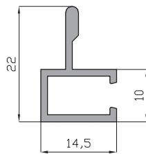
Marco perfil mosquitera 54570
