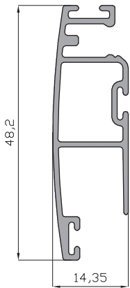
Perfil mosquitera Curvo 14320
