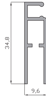
Perfil mosquitera 1492
