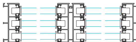
Sección Vertical
