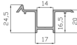
Guía Inferior Plegable Cala 16565
