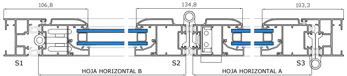
Sección horizontal de 2 hojas cerradas
