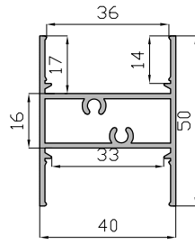
Zócalo de 50 MM 14723
