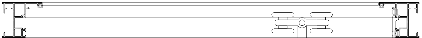
Sección horizontal de 3 hojas abiertas
