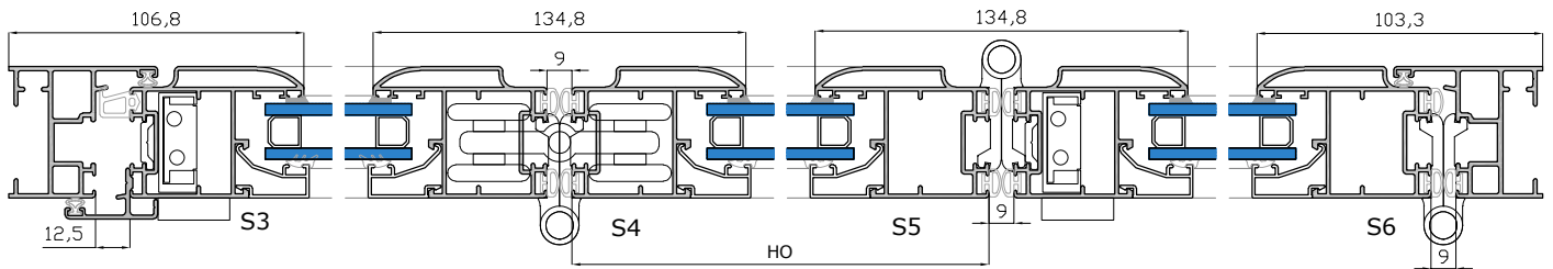
Sección horizontal de 3 hojas cerradas
