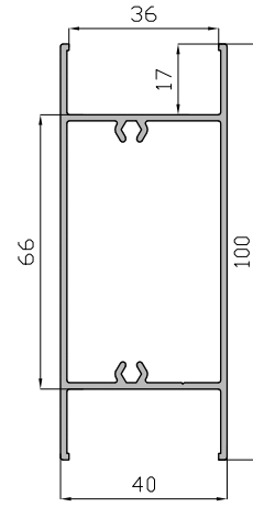
Zócalo de 100 mm 15610
