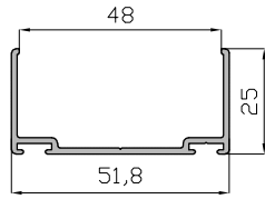
Compensador Plegable Cala 16564
