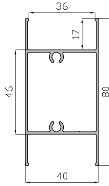
Zócalo de 80 MM 18901
