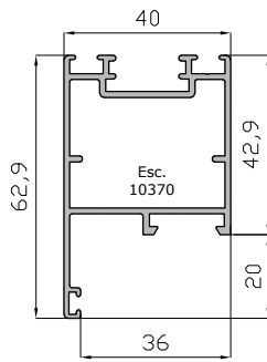
Hoja Acristalar Plegable 16566
