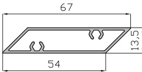
Lama Romboidal Autorroscada 12846
