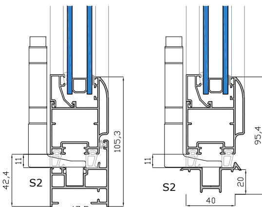
Sección Vertical Guía inferior embutida
