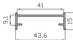
Base Lama Troquelada 15441
