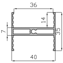
Divisor Mallorquina 35 MM 18311
