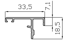
Perfil Cierre Plegable Cala 16568
