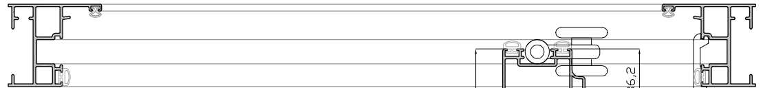
Sección horizontal de 2 hojas abiertas
