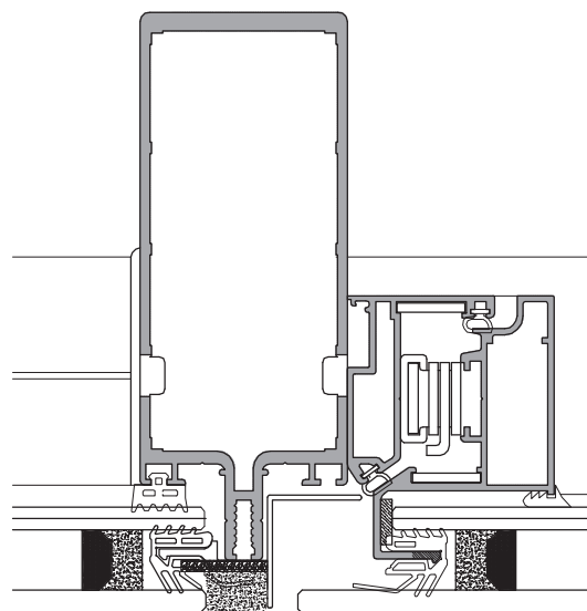
SISTEMA ESTRUCTURAL DIRECTO
