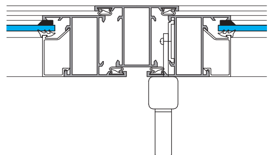
Sección horizontal 2 hojas
