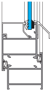
Sección Vertical
