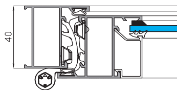
Sección horizontal 2 hojas
