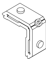
Escuadra Ventana (Hoja perimetral + Fijos RPT) 82110
