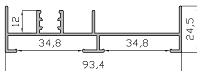
Marco Lateral Recto 5931
