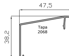
Cumbrea 47.5 mm 14655
