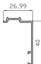
Solape 40 mm 5563
