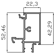
Esquinero 90° 14661
