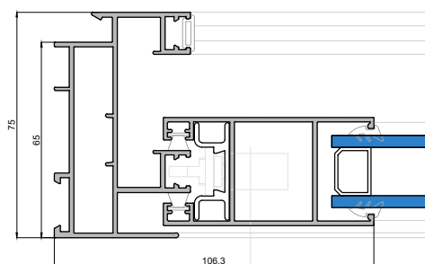
Sección Horizontal
