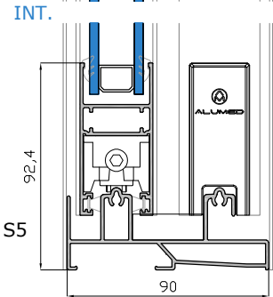
Sección Vertical
