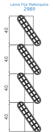
Detalle Sección de la lama
