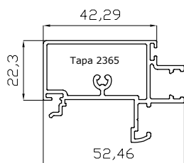
Esquinero 90° 14661
