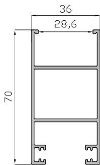
Hoja Lateral 14648
