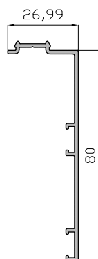
Solape 80 mm 5564
