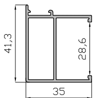
Hoja Central Ventana 17629
