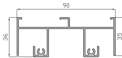
Marco Superior Recto 5932
