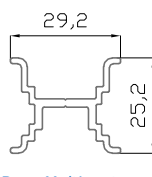
Base Multipunto hoja perimetral PVC 15578
