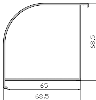
Esquinero 90° 12263
