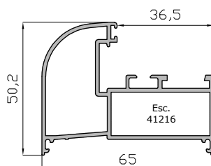
Marco Fijo 65 mm. Alumed 40 18241
