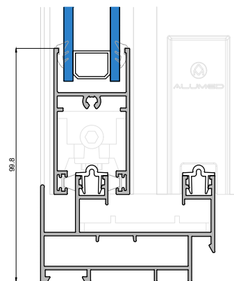
Sección Vertical
