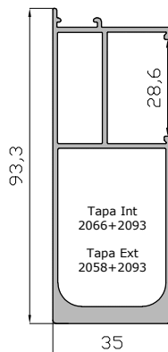
Hoja Central Reforzada 17858
