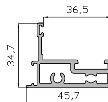
Cruce Monocarril Unicarril 5973
