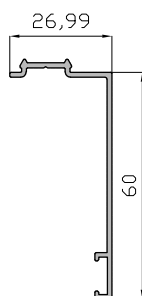
Solape 60 mm 5678
