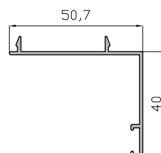
Solape 40 Marcos Rectos 5935
