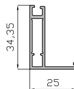
Hoja Central Reducida Ventana 17627
