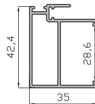
Hoja Central Ventana 15629
