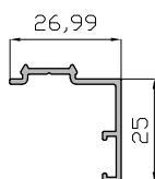
Solape 25 mm 5562
