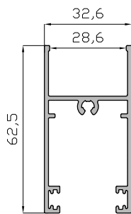
Hoja Rueda 14649
