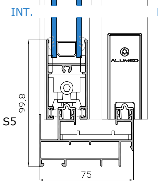
Sección Vertical
