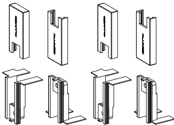
Kit Hoja Central Reducido (17626 y 17627) 2097
