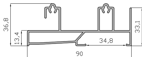
Marco Inferior Recto 5933
