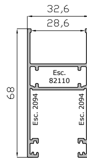
Hoja Perimetral 17940
