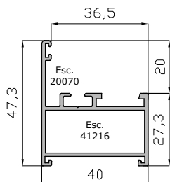
Marco Ventana 40 mm 17034
