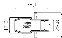
Unión 4 hojas 15854
