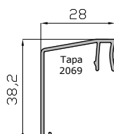
Cumbrea 28 mm 14654
