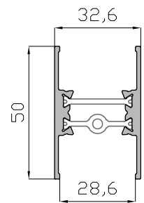
Divisor Hoja RPT 5419
