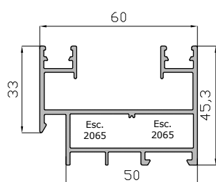
Marco Prmt 60 mm 14646
