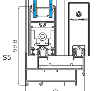
Sección Vertical
