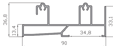
Marco Inferior Recto 5933
