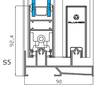
Sección Vertical
