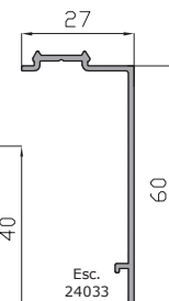
Solape 60 mm 5678
