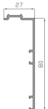
Solape 80 mm 5564
