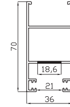
Mecanizado Multipunto Lateral Hoja Lateral RPT REF: 14648 (comprobar medidas)
