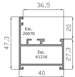
Marco Ventana 40 mm 17034
