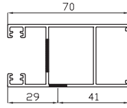
Mecanizado Multipunto Lateral Hoja Lateral RPT REF: 14648 (comprobar medidas)
