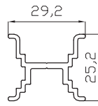
Base Multipunto hoja perimetral PVC 15578
