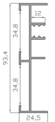
Marco Lateral Recto 5931
