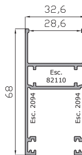
Hoja Perimetral 17940
