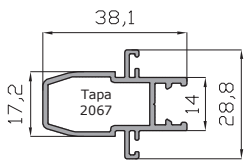
Unión 4 hojas 15854
