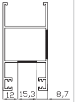
Mecanizado Multipunto Lateral Hoja Lateral RPT REF: 14648 (comprobar medidas)
