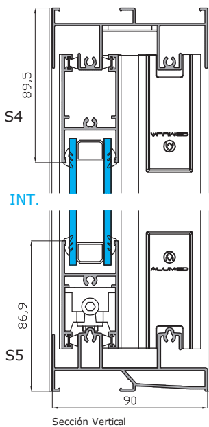
Sección Vertical
