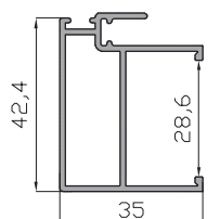
Hoja Central Ventana 15629
