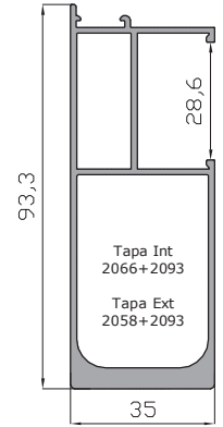
Hoja Central Reforzada 17858
