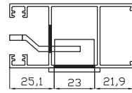
Mecanizado Multipunto Lateral Hoja Lateral RPT REF: 14648 (comprobar medidas)
