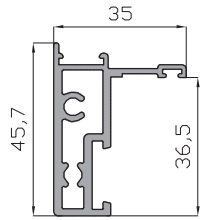
Cruce Monocarril Unicarril 5973
