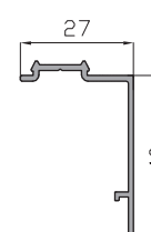
Solape 40 mm 5563
