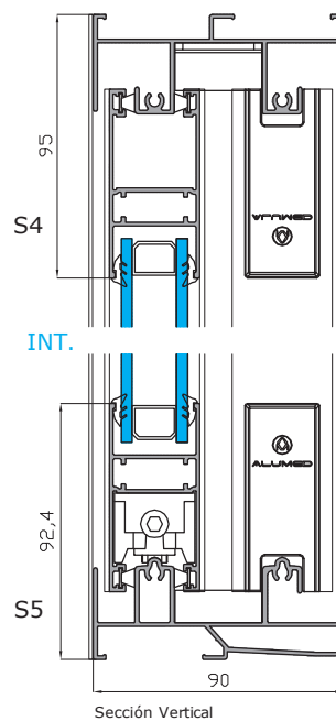
Sección Vertical
