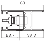
Mecanizado Multipunto Hoja perimetral REF: 17940 (comprobar medidas)
