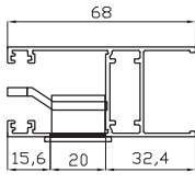
Mecanizado Cierre Embutido Hoja perimetral REF: 17940 (comprobar medidas)
