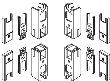
Kit Technica 2 hojas Perimetral 2192
