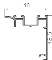
Cruce Hoja Centro Perimetral 17938
