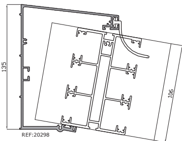
- TECHO FIJO 3 CARRILES
