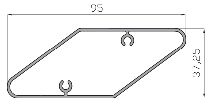
Lama romboidal autorroscada 18315
