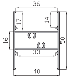
Zocalo de 50 MM 14723
