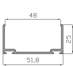
Compensador plegable cala 16564
