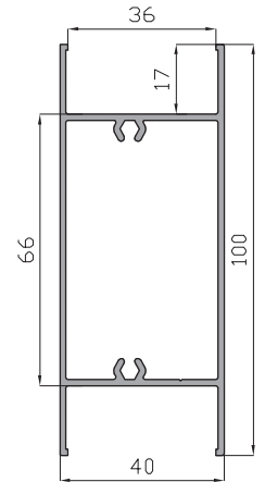
Zocalo de 100 mm 15610
