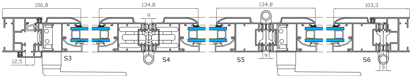
Sección horizontal de 3 hojas cerradas
