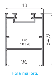
Hoja mallorq. plegable cala 16567
