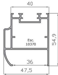
Hoja curva mallorq. plegable cala 15679
