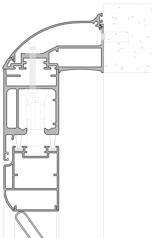
Sección Vertical
