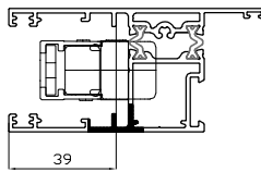
Mecanizado Elevable HS200 Hoja perimetral REF: 15696 Ver documentación del herraje (comprobar medidas)
