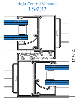
S1 Tipología de Nudos Centrales
