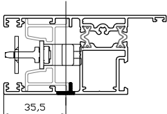
Mecanizado Multipunto Hoja perimetral REF: 15696 (comprobar medidas)
