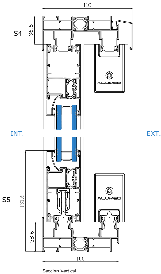
Sección Vertical
