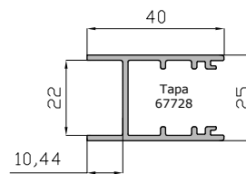
Unión 4 Hojas Elevable 15573
