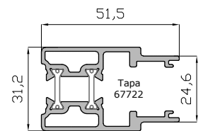
Unión 4 Hojas RPT 15695
