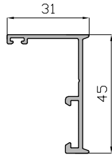
Acople Junquillo Hoja Recta 5433
