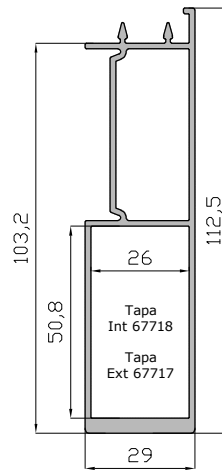
Hoja Central Reforzada 15432
