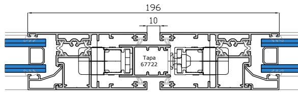
Corte 15573 = Altura de la hoja - 45 mm
