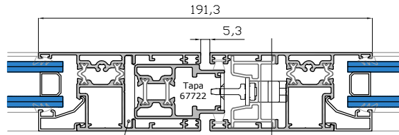
Corte 15695 = Altura de la hoja - 70 mm
