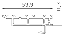
Cruce Hoja Prmt PVC 15562
