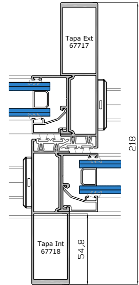
Hoja Central Reforzada 15432
