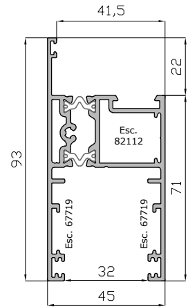
Hoja Perimetral RPT 15696
