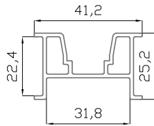
Base Multipunto PVC 15572
