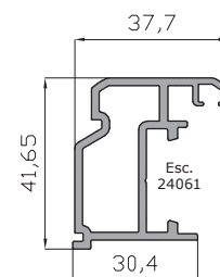
Inversor A58 85805
