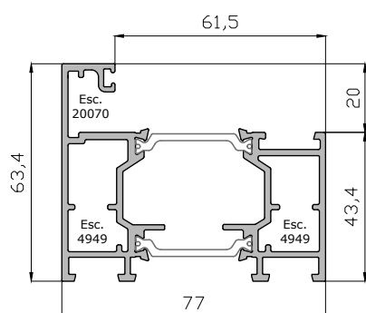
Hoja Plegable 12432
