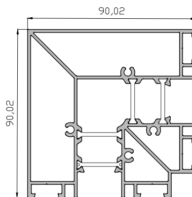
Esquina 90° 12444
