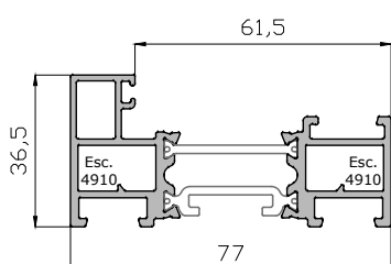
Hoja Minimalista 12442
