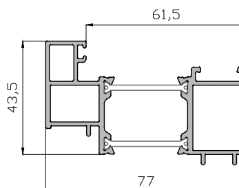
Hoja Minimalista Comp. Cerradura 12443
