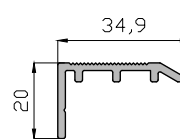
Solape Antideslizante 12435
