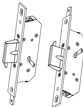
Kit Desviad. Falleba Cerradura 49230
