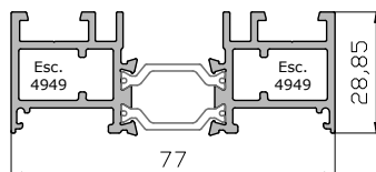
Marco Plegable Sin Ala 12431
