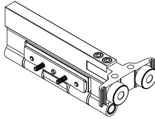
Bisagra Patín Superior 4943
