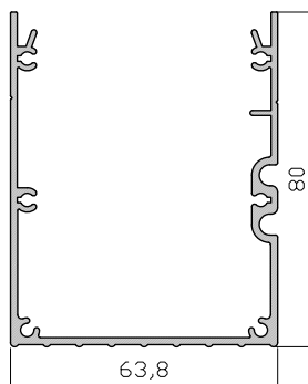
Canal 12407
