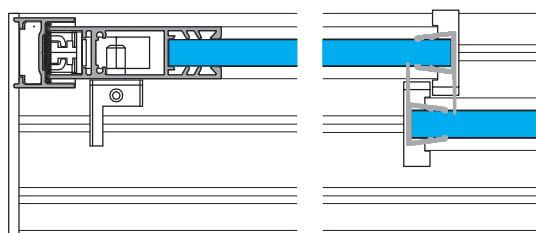
Sección horizontal
