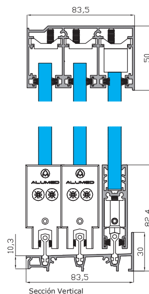
Sección Vertical
