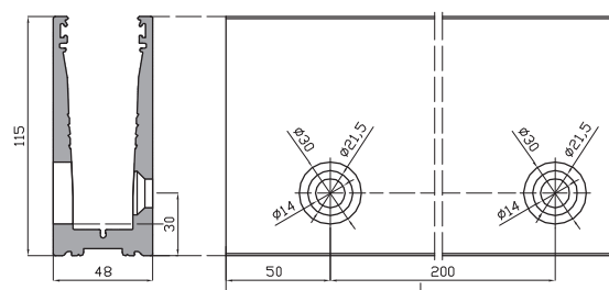
Pefil U 54300-MF03
