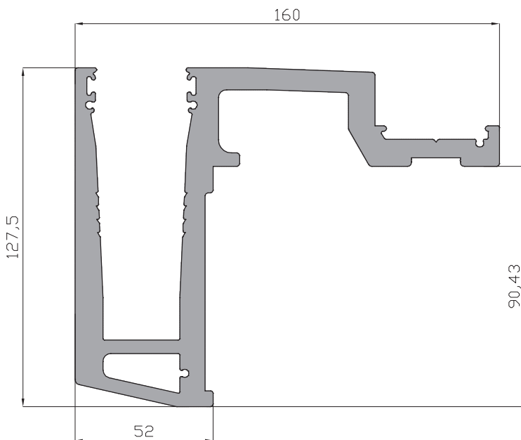
Perfil U.L. Frontal 54303
