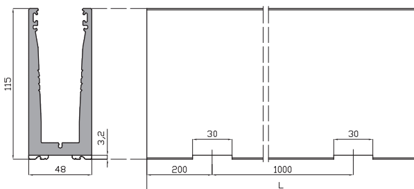
Pefil U 54300 MD-01
