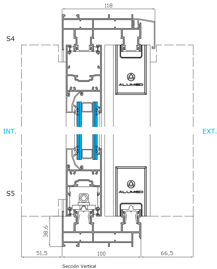
Sección Vertical
