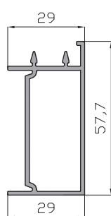
Hoja Central Ventana 15431
