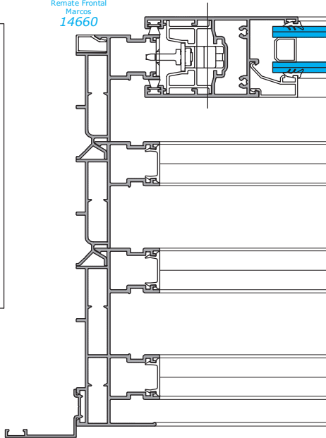
S2 Acople Pluricarril y solape
