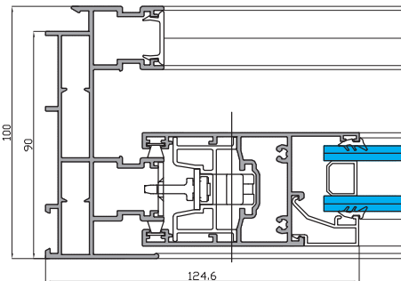
Sección Horizontal
