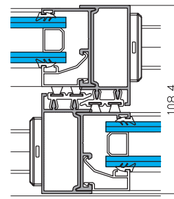
S1 Tipología de Nudos Centrales
