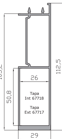
Hoja Central Reforzada 15432
