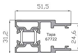
Unión 4 Hojas RPT 15695
