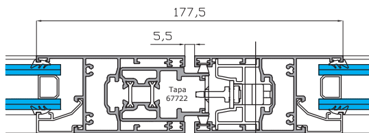
S4 Unión 4 hojas
