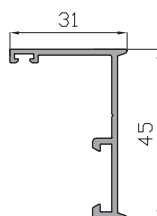
Acople junquillo hoja recta 5433
