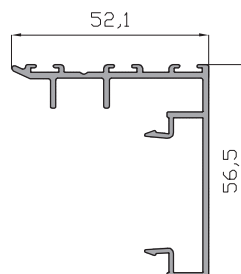
Cruce hoja Perimetral 5573
