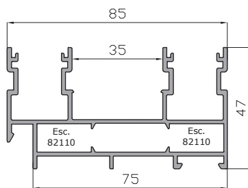
Marco Perimetral 85 mm. 5604
